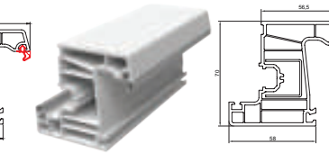
DÜZ KANAT PROFİLİ
