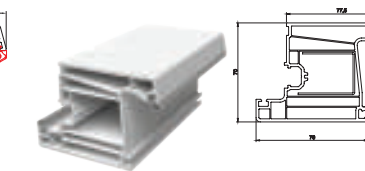
İÇE AÇILIR KAPI PROFİLİ
