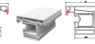
DIŞA AÇILIR KAPI PROFİLİ
